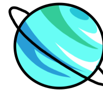
planet
